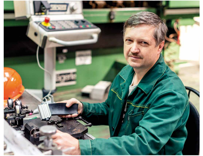
Изготовление рабочей лопатки ГТК-10-И на заводе «Турбодеталь»
