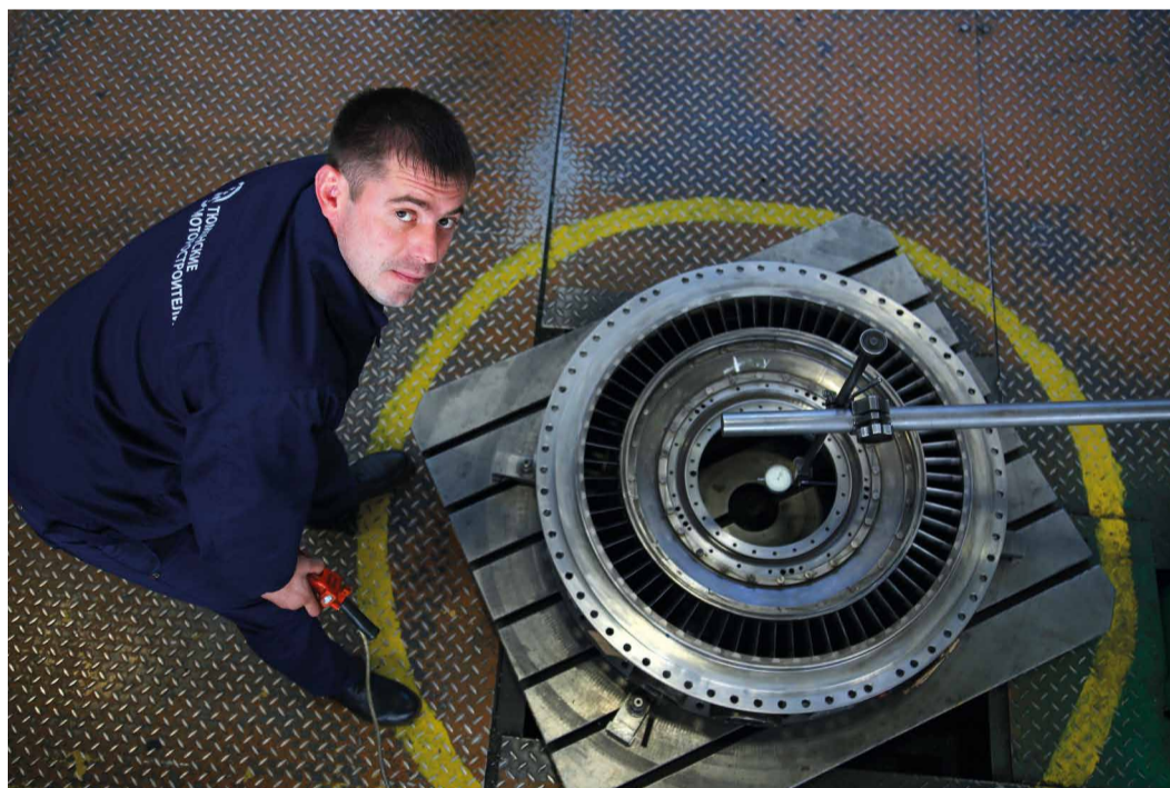
Этап центровки корпусных деталей газотурбинного двигателя в цехе ПАО «ТМ»
