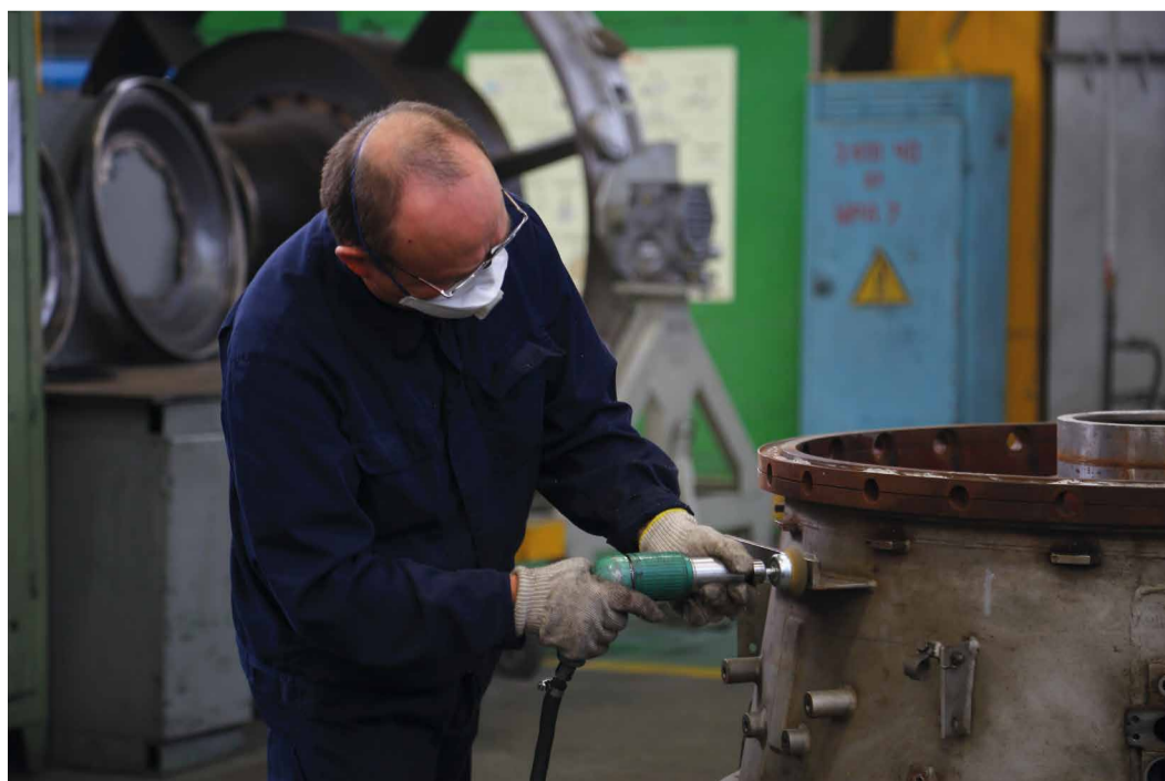
Сотрудник ПАО «ТМ» зачищает поверхность от коррозии
