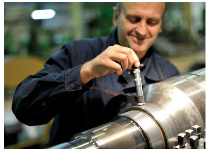
Рабочий завода «Турборемонт» выполняет контроль изготовления вала ротора
