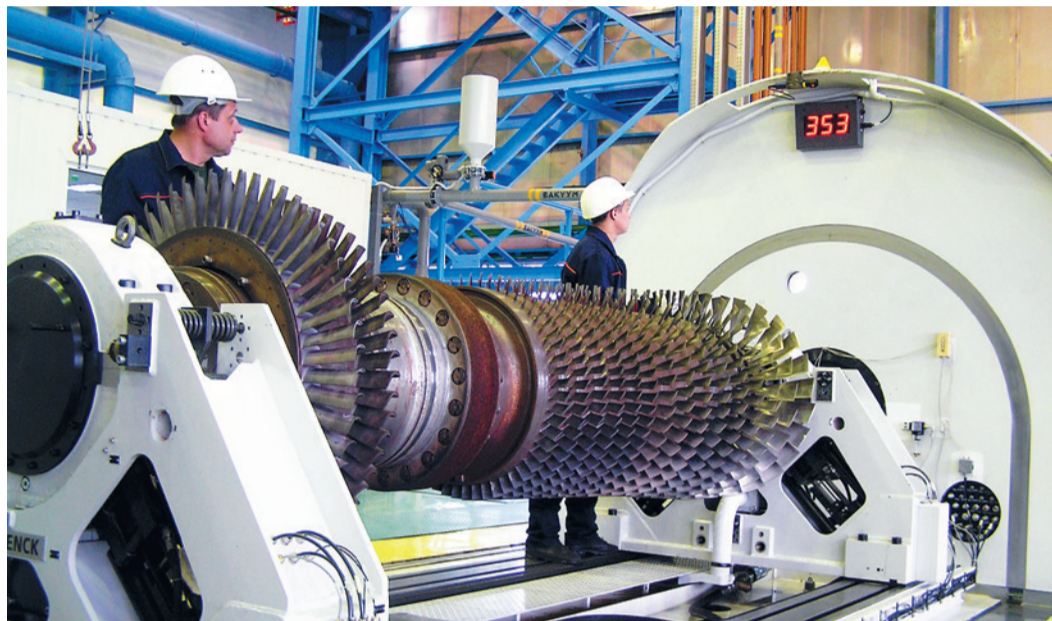
Разгонно-балансировочный стенд
